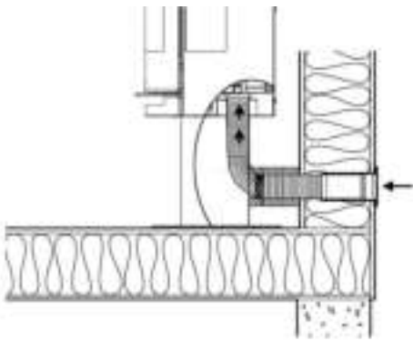
À travers le mur
