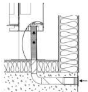
Via golv och fundament
