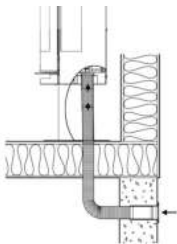
Via golv och krypkällare
