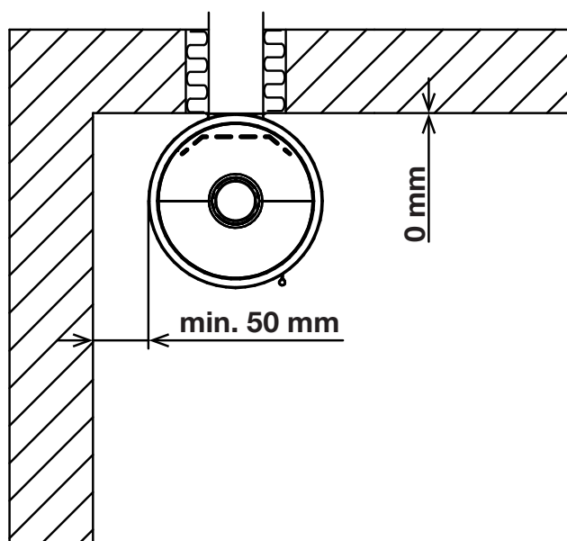
Stěna z nehořlavého materiálu
