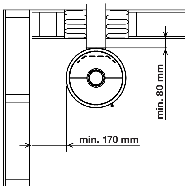
Stěna z hořlavého materiálu
