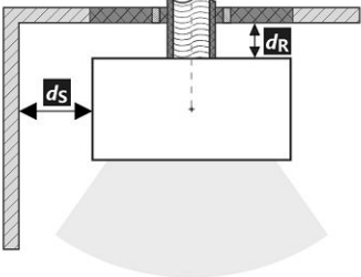
Заднее подключение дымохода (изолированное)
