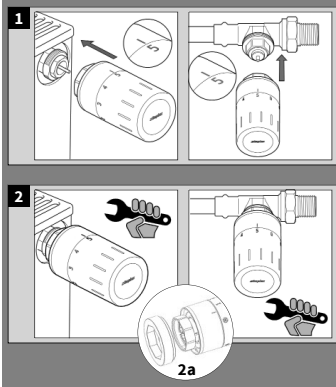
Závitová přípojka M30 × 1,5 Závitová prípojka M30 × 1,5
