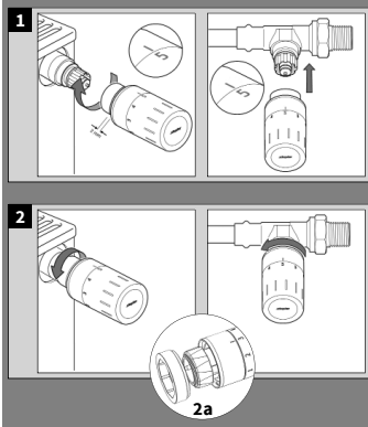
Svěrná přípojka Zverná prípojka
