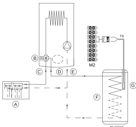
Obr. 96 Pripojenie zásobníka TUV
