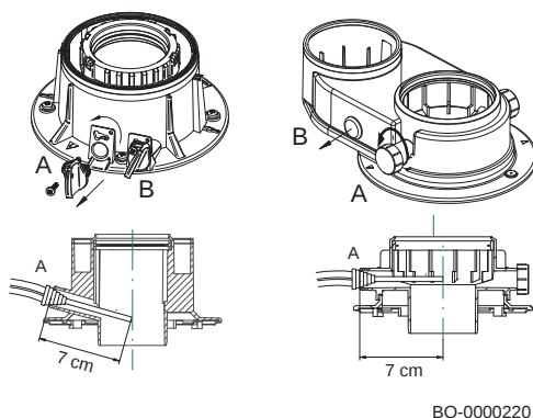
Obr. 50 Typ připojení - měřicí přípojka pro spaliny
