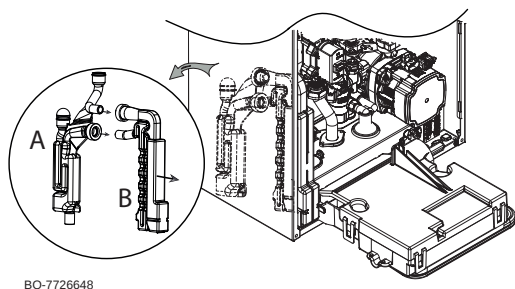
Obr. 131 Demontáž sifónu
