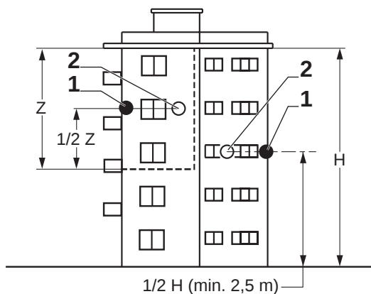
Obr. 27 Doporučená umístění A
