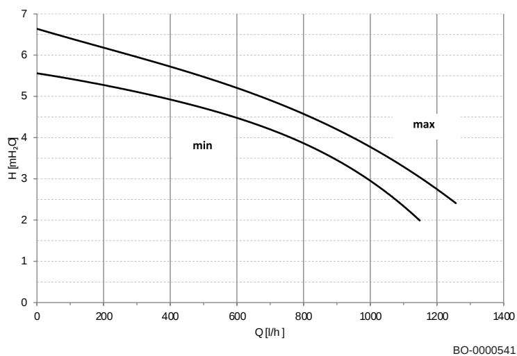
Obr. 88 Graf zostatkového výtlaku predimenzovaného čerpadla ( kúrenie + kotol na TÚV )
