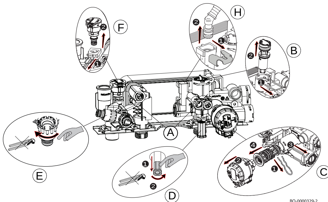
Obr. 133 Časti kúrenia + TÚV kombinovanej jednotky kotlovej vody
