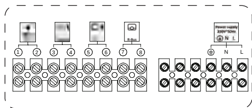
Obr. 109 Pripojenia dosky kotla
