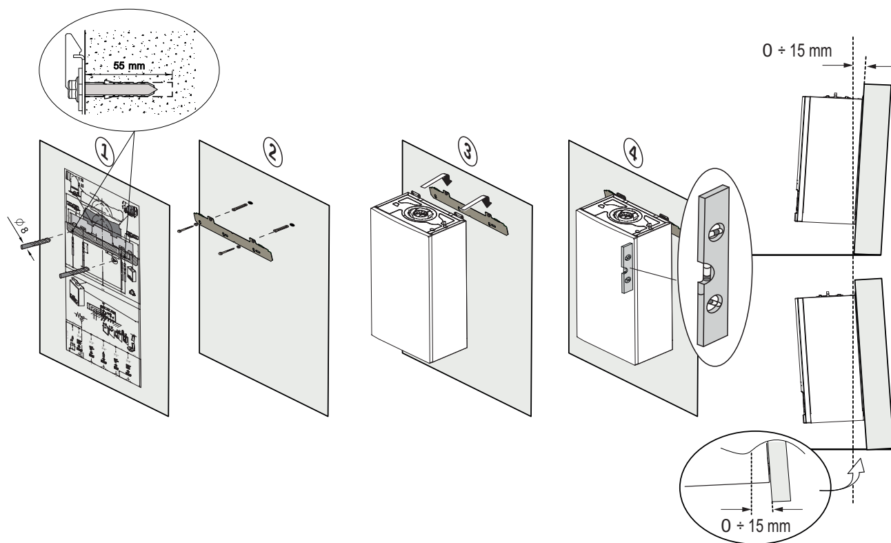
Obr. 93 Inštalácia na stenu
