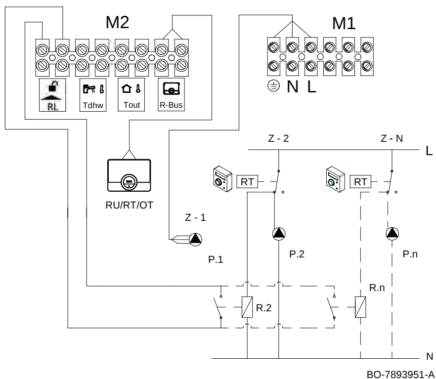
Obr. 45 Příklad instalace s relé
