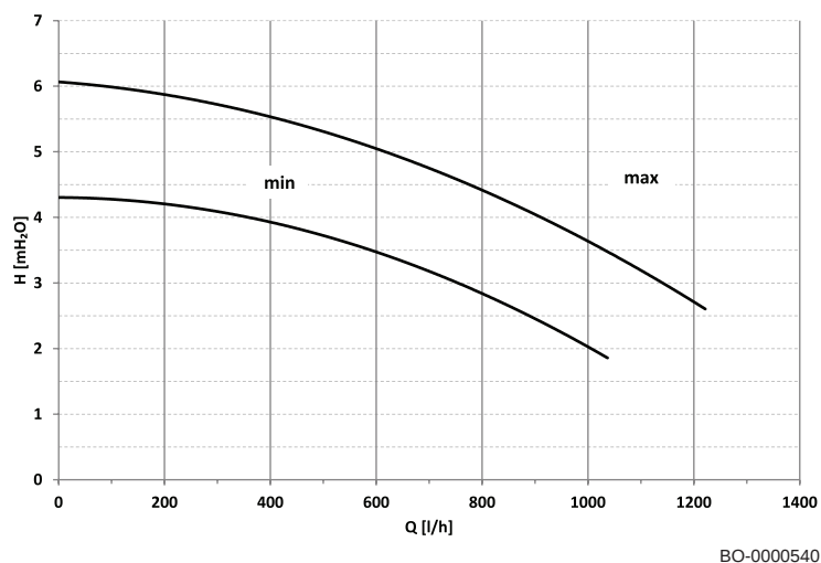
Obr. 88 Graf zostatkového výtlaku predimenzovaného čerpadla ( kúrenie + kotol na TÚV )
