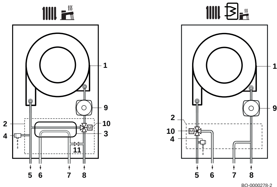
Obr. 82 Schematický diagram
