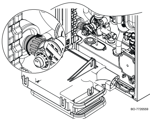
Obr. 115 Vypúšťanie vykurovacieho systému
