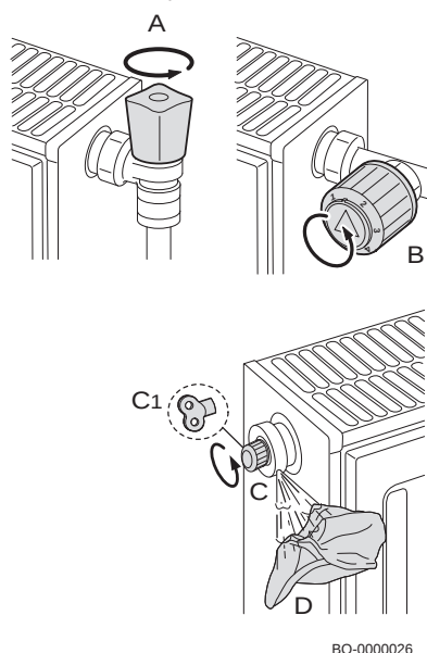
Obr. 78 Čistenie systému
