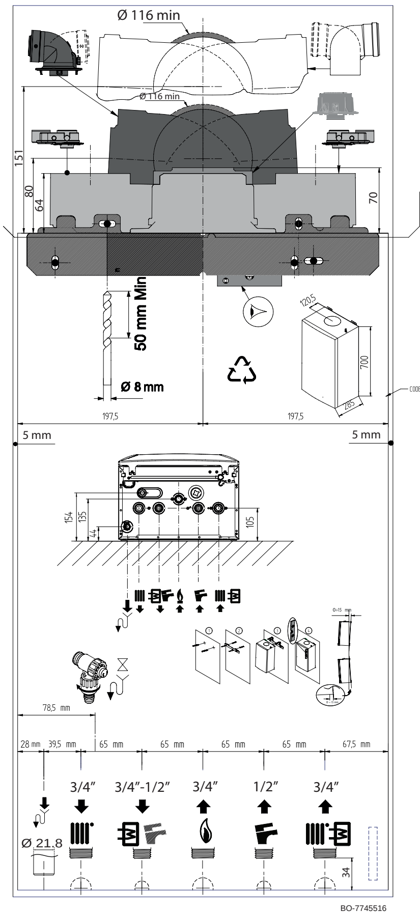
Obr. 80 Papierová šablóna kombinovaného modelu Vykurovanie + Teplá úžitková voda
