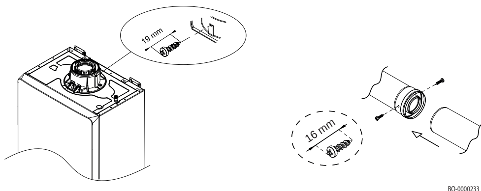
Obr. 33 Upevnění věže koaxiálního odvodu spalin
