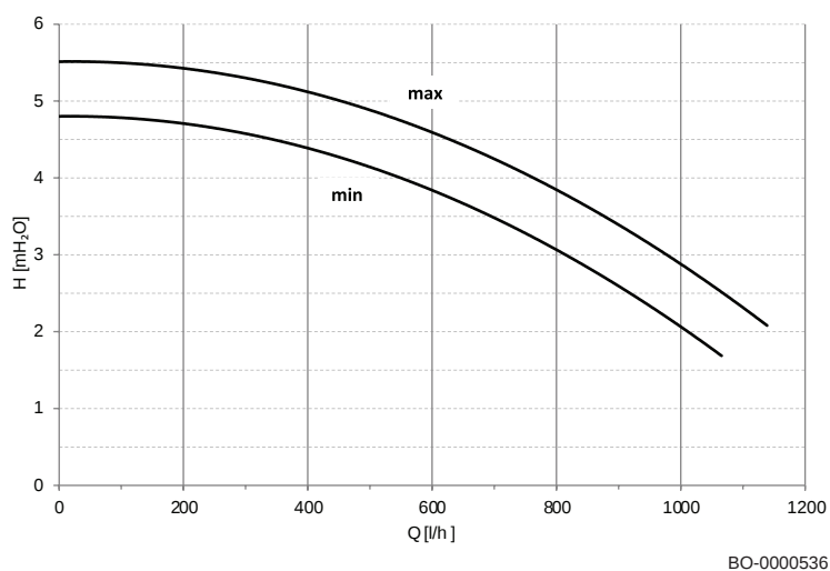
Obr. 86 Graf zostatkového výtlaku čerpadla ( kúrenie + kotol na TUV )
