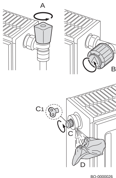
Obr. 11 Čištění soustavy
