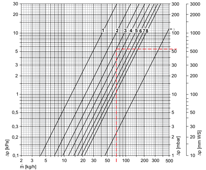
Ventilová vložka VHV8S s 8 stupni nastavení
