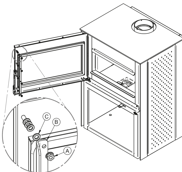
Obrázek 18: Nastavení západky dvířek
