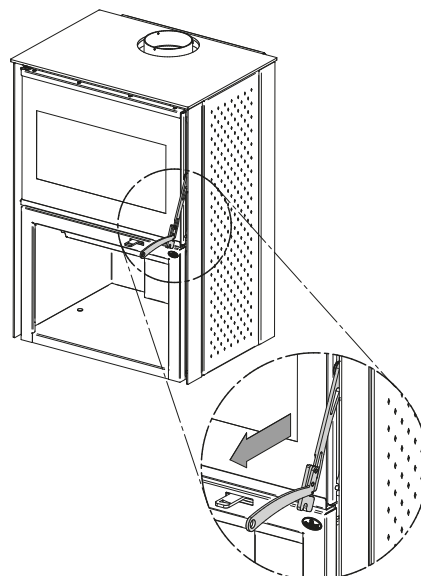
Obrázek 9: Zatáhněte za studenou rukojeť a otevřete dvířka
