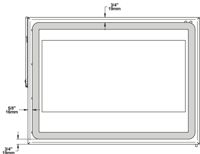
Obrázek 16: Výměna těsnění skla
