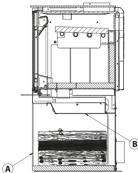
Obrázek 12: Skladování polen pod kamny
