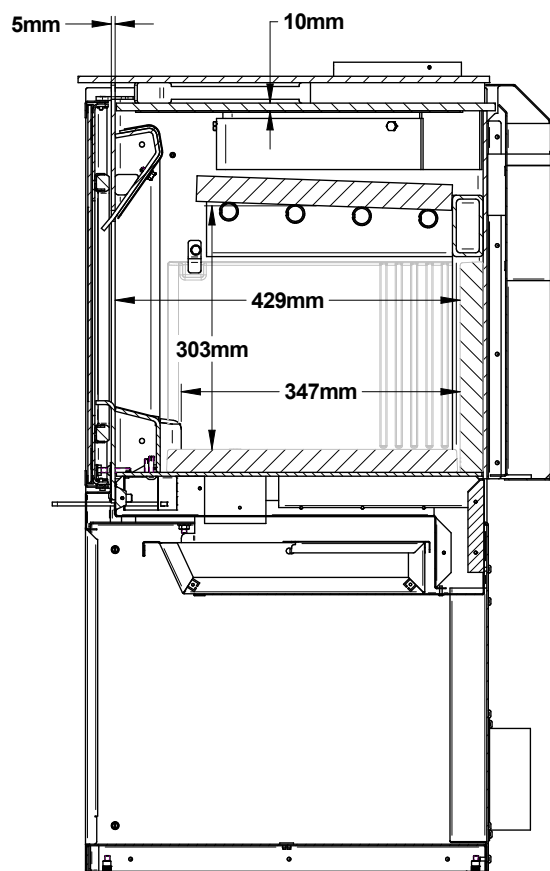
Obrázek 6: Pohled z boku – spalovací komora
