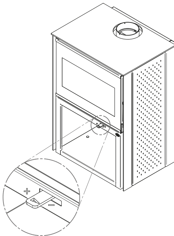
Obrázek 13: Ovládání přívodu vzduchu
